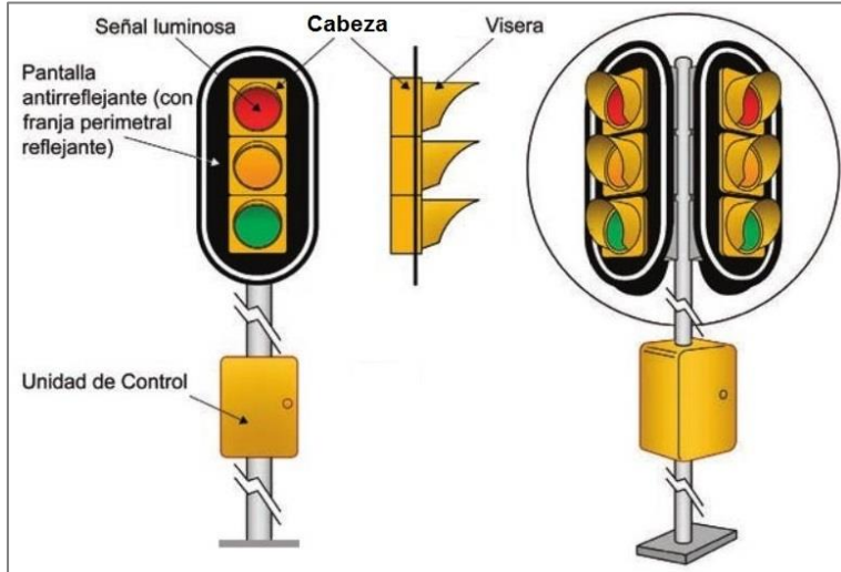
Figura 6.3 Ejemplo de configuración de cabeza de semáforos
