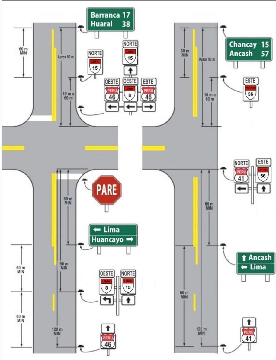
Figura 2.29 Ejemplo de conjunto de indicadores de ruta
