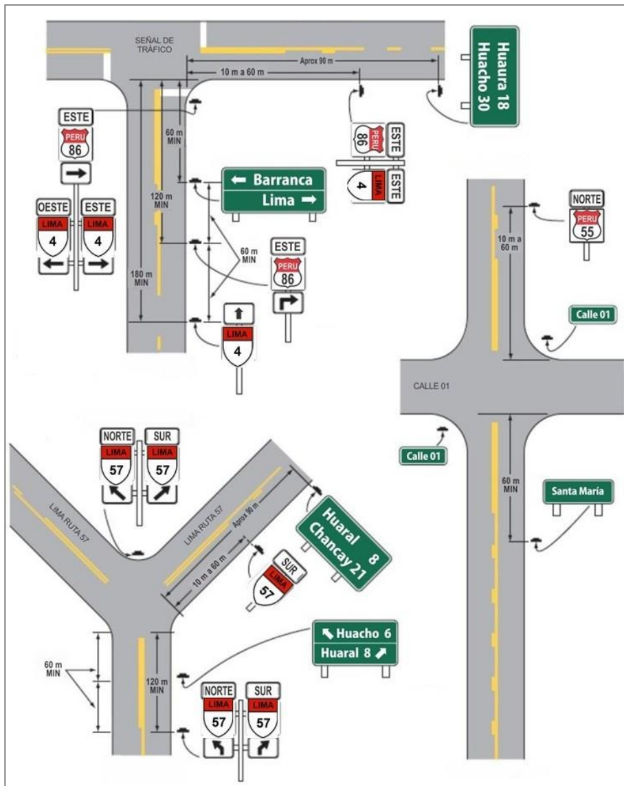
Figura 2.30 Ejemplo de conjunto de indicadores de ruta
