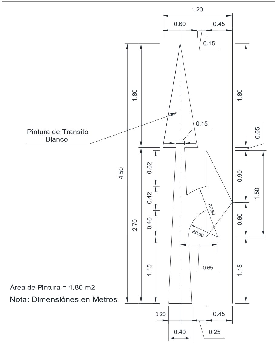
Figura 3.47 Dimensiones de combinación de flecha recta y de giro
