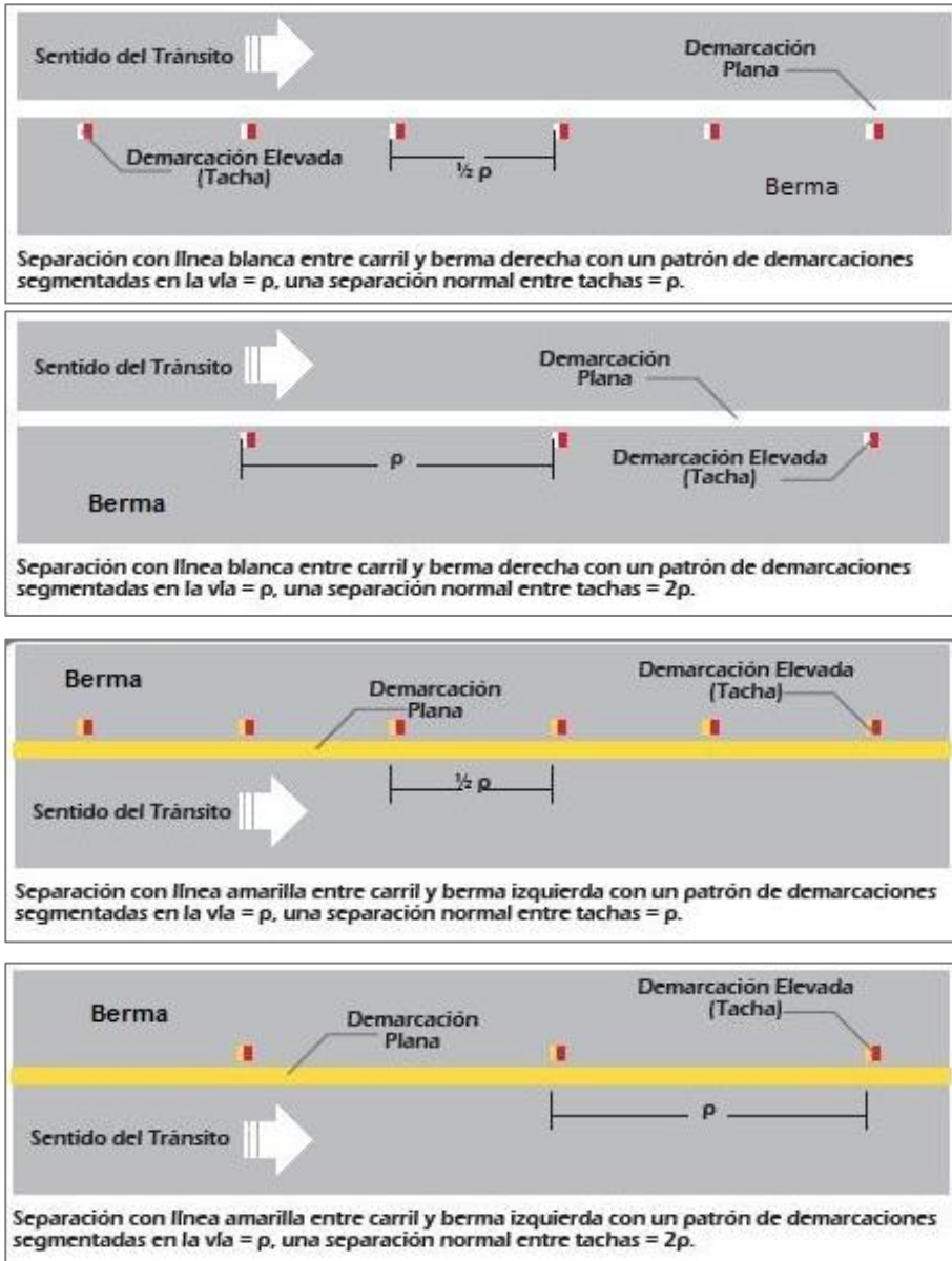
Figura 3.3 Ejemplos de línea de borde de calzada o superficie de rodadura
