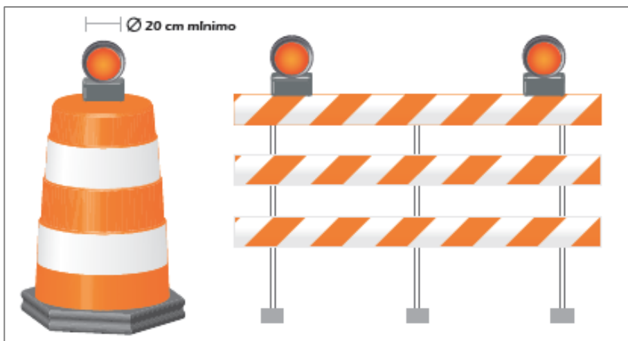
Figura 5.9 Ejemplo de barreras reforzadas con dispositivos luminosos.
