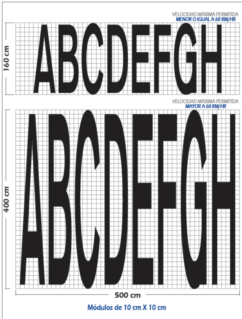
Figura 3.53 Dimensiones de la demarcación de leyenda
