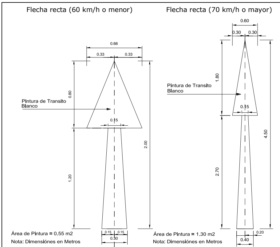
Figura 3.43 Dimensiones de flecha recta
