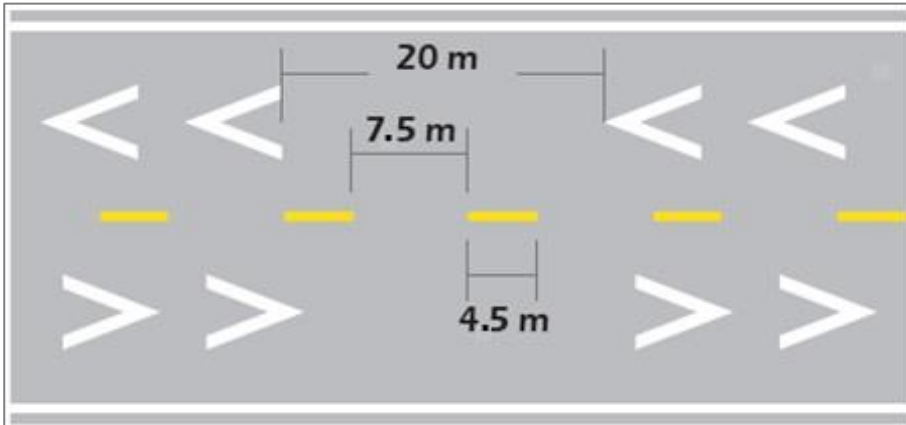
Figura 3.39 Ejemplo de demarcación de "DISTANCIADORES"
