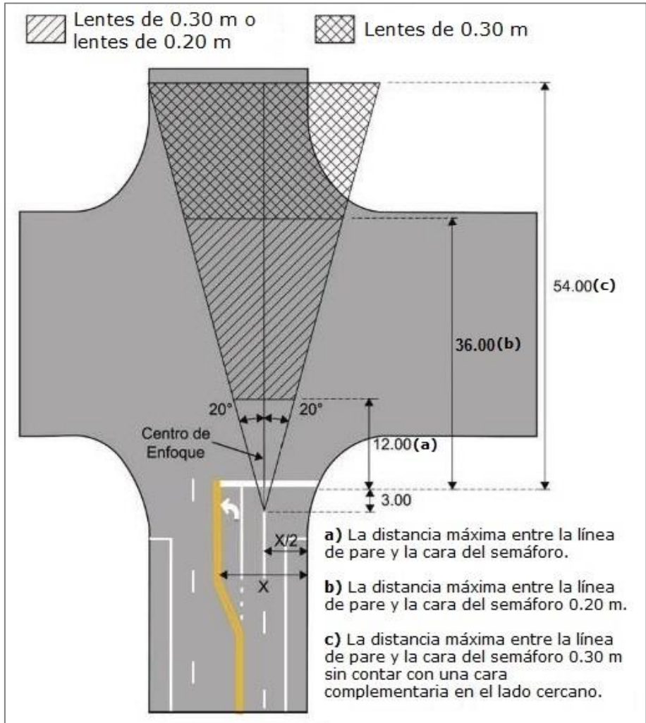
Figura 6.6 Ejemplo de ubicación de las caras de un semáforo en el lado más lejano del acceso a la intersección
