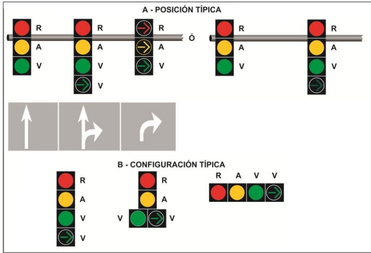
Figura 6.32 Ejemplo de disposición de indicadores de semáforos con giros a la derecha protegidos sin carril de giro exclusivo
