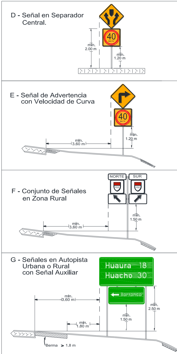
(Continúa) Figura 2.5 Ejemplo de Ubicación Lateral
