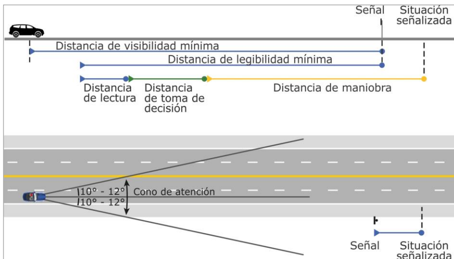
Figura 2.4 Ubicación Longitudinal y Distancias de Lectura
