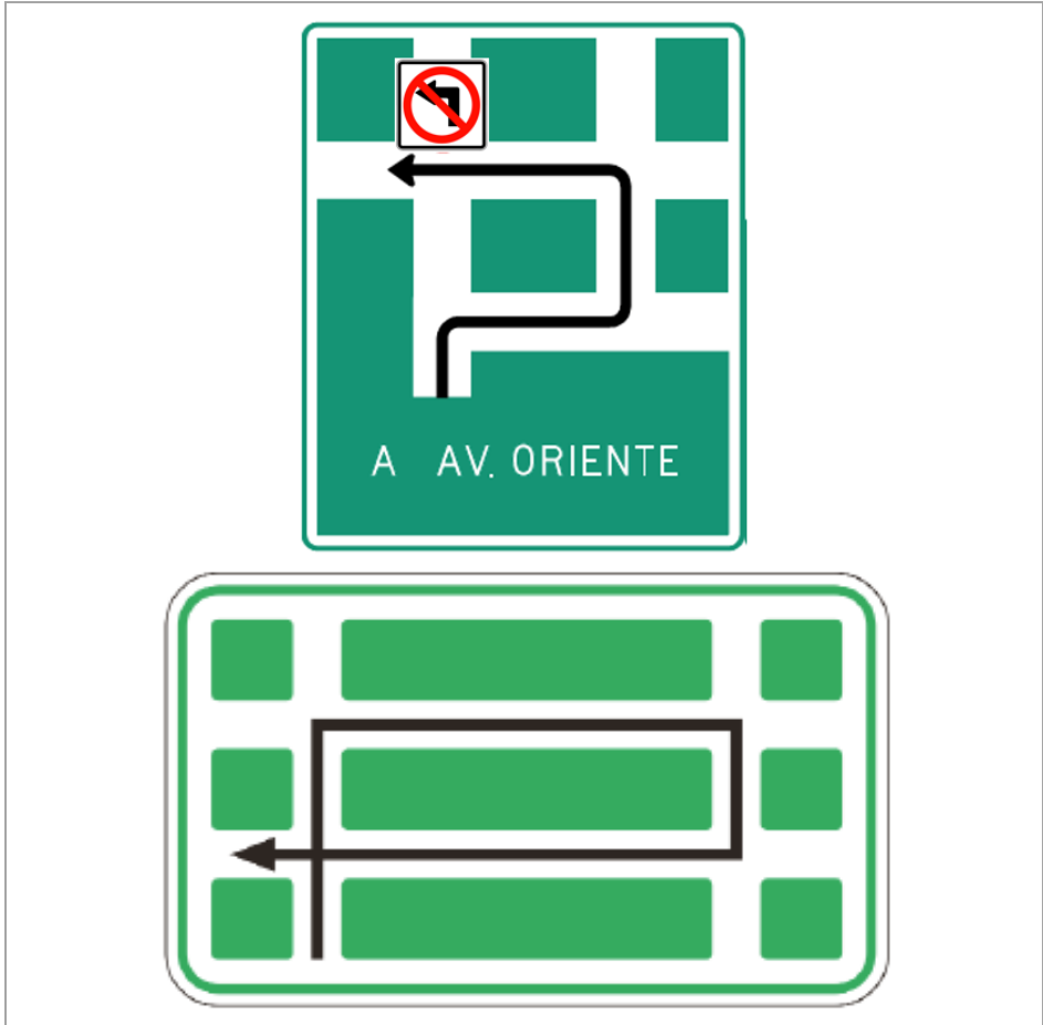
Figura 2.31 Ejemplos de diagramación de pre señalización en intersecciones o cruces en zonas urbanas con limitación de giro
