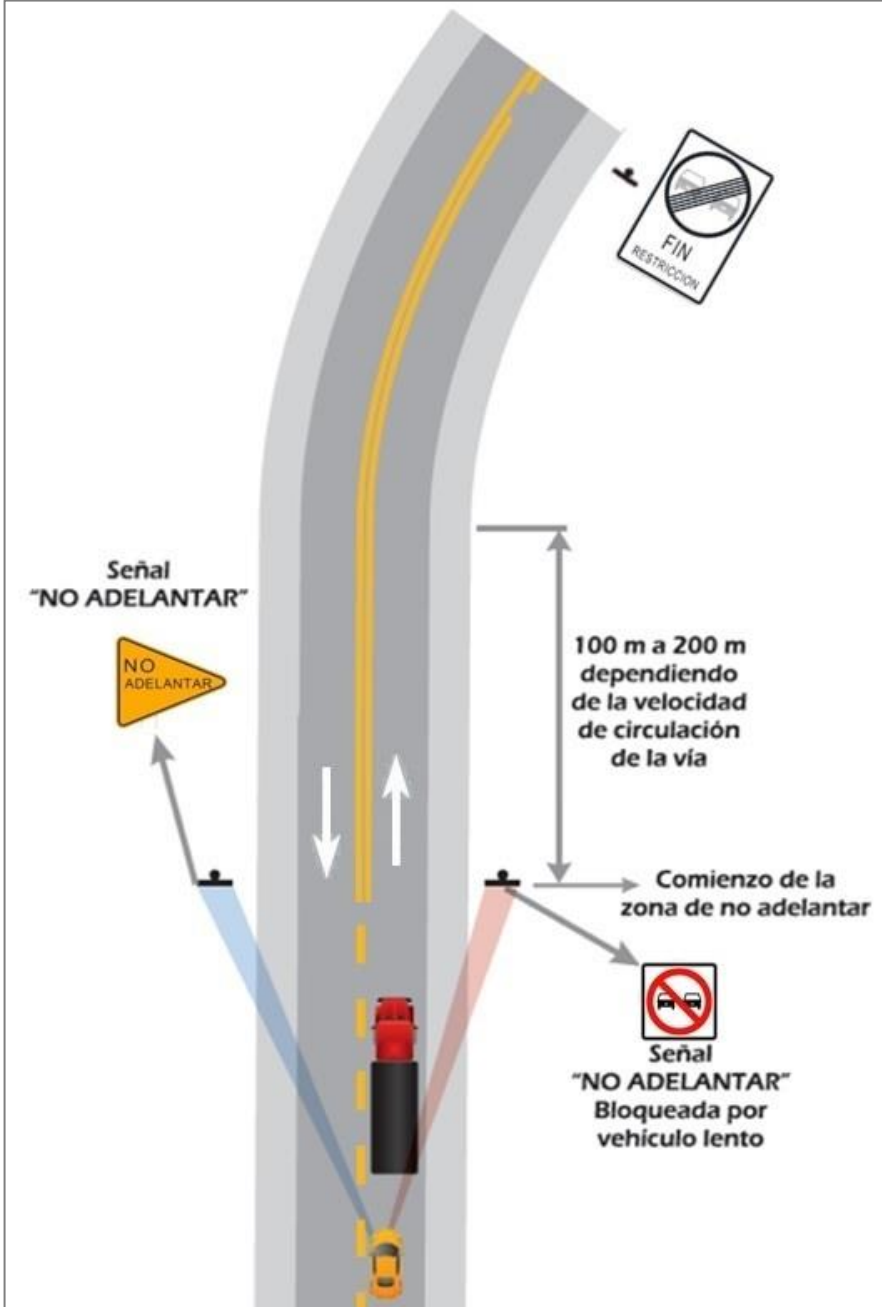
Figura 3.10 Ejemplo de zona o tramo con prohibición de adelantamiento complementado con señalización vertical
