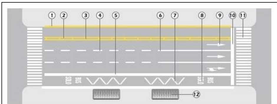
Figura 3.18 Ejemplo de demarcación de paraderos de buses
