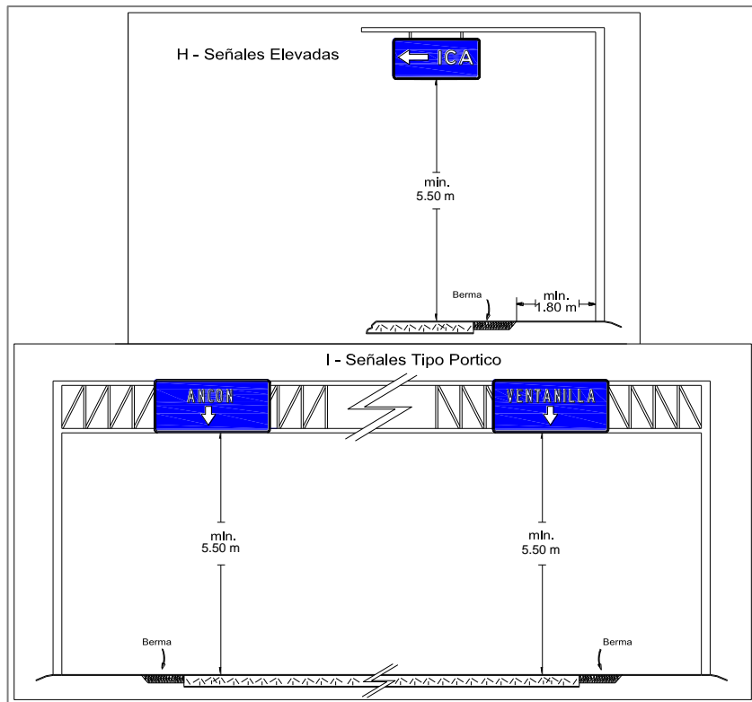
(Continua) Figura 2.5 Ejemplo de Ubicación Lateral
