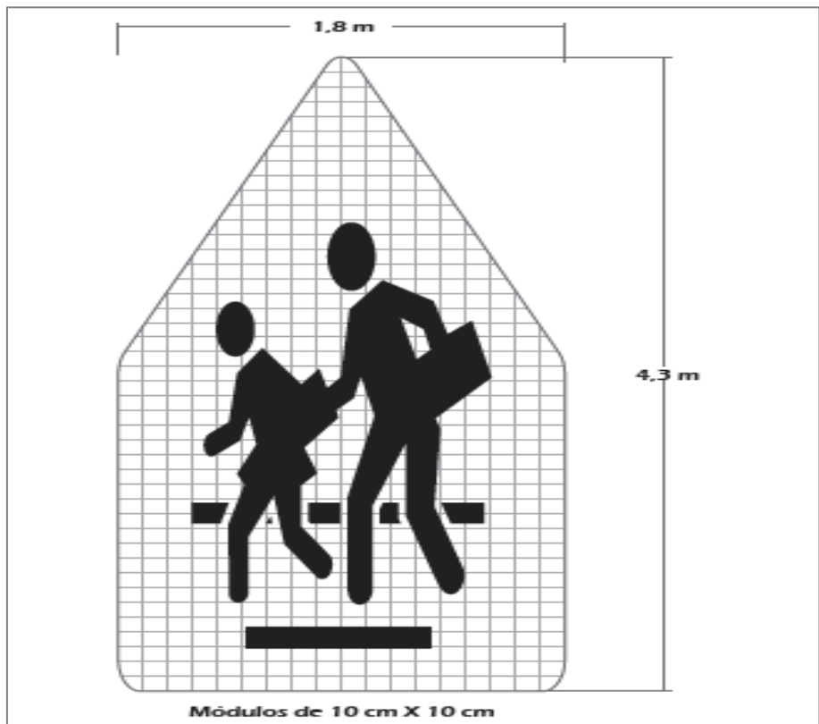
Figura 3.38 Dimensiones de demarcación "ZONA ESCOLAR"
