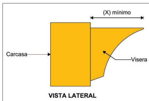
Figura 6.11 Ejemplo de visera de semáforo
