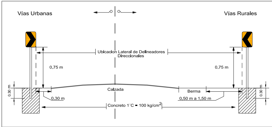
Figura 3.63 Ejemplo de ubicación de delineadores "CHEVRON"
