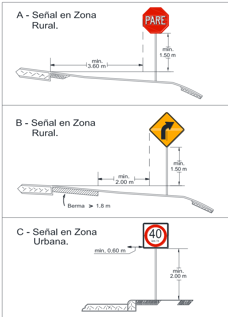
Figura 2.5 Ejemplo de Ubicación Lateral
