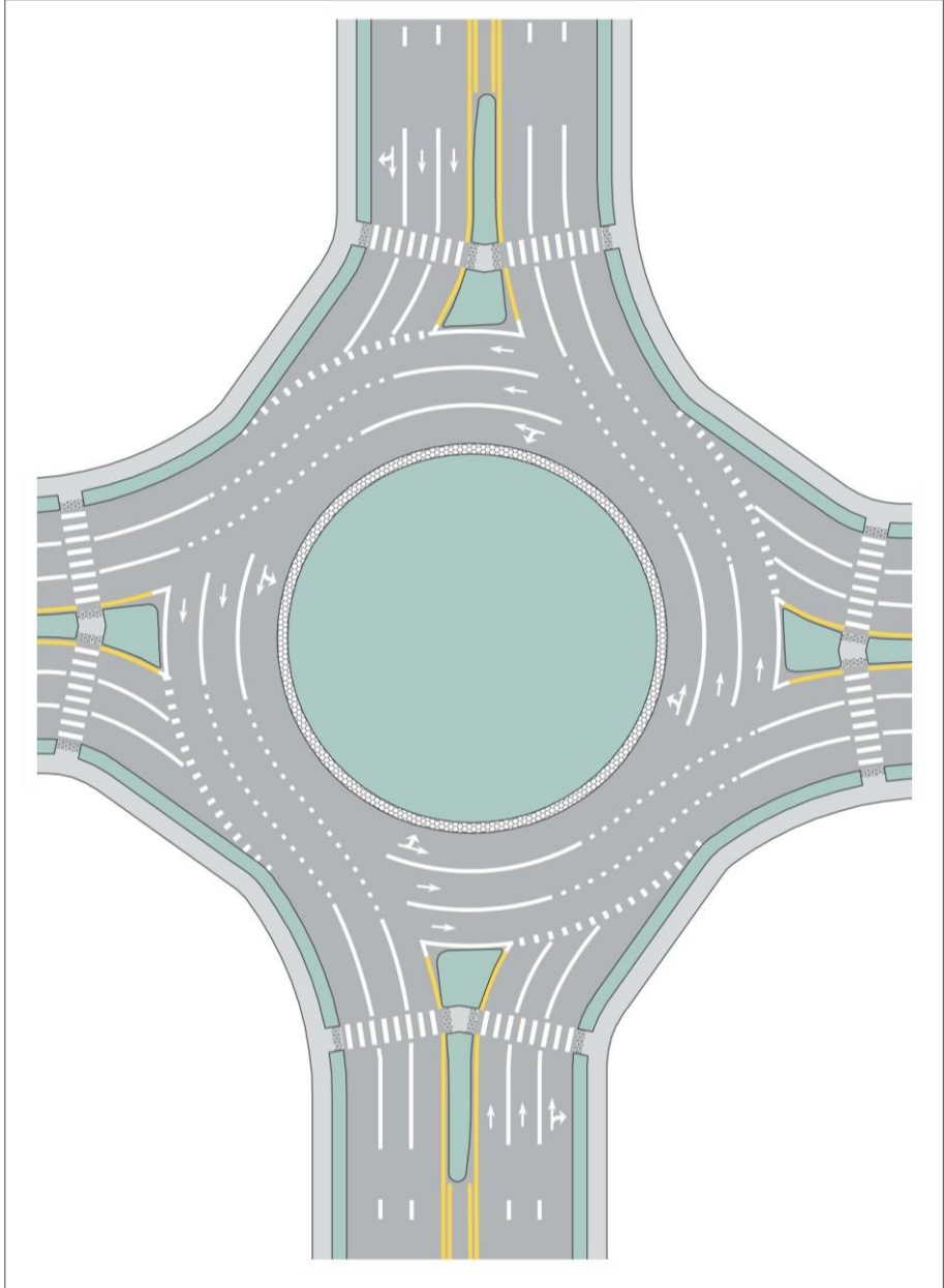
Figura 3.30 Ejemplo de demarcación para intersecciones tipo Rotonda o Glorieta de tres carriles con tres carriles de acceso
