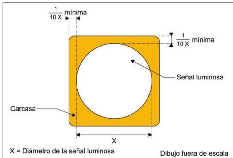
Figura 6.8 Ejemplo de modulo luminoso de un semáforo
