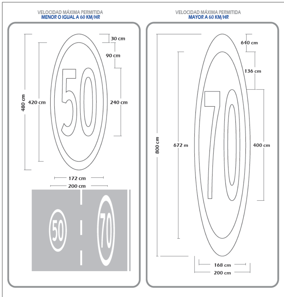
Figura 3.35 Dimensiones de demarcación "VELOCIDAD MÁXIMA PERMITIDA"
