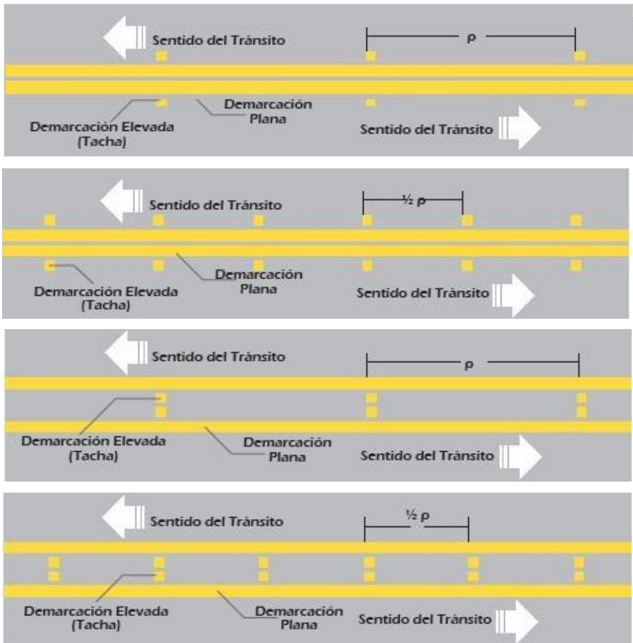
Figura 3.8 Ejemplos de línea continua doble
