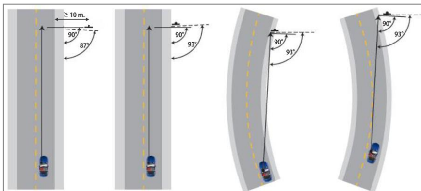
Figura 2.6 Ejemplo de Orientación de la Señal
