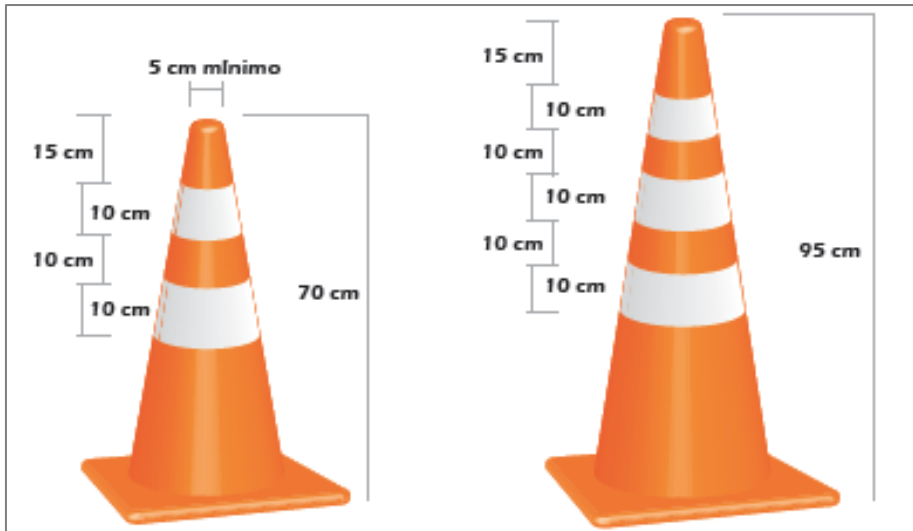
Figura 5.3 Ejemplo de conos con dimensiones
