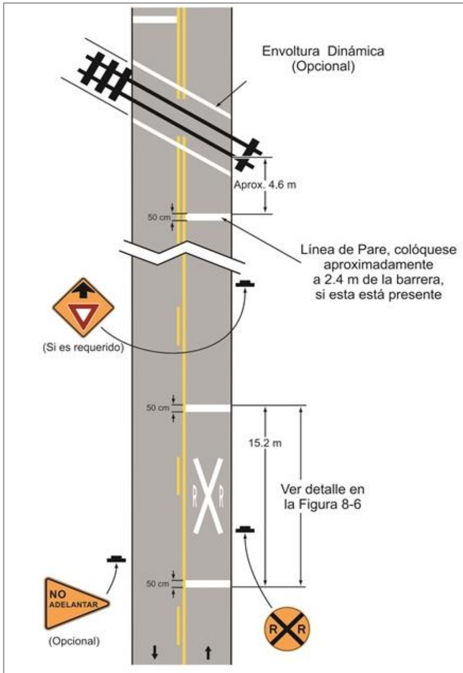
Figura 4.15 Ejemplo de señalización vertical y horizontal y dimensiones, en un cruce ferroviario a nivel oblicuo
