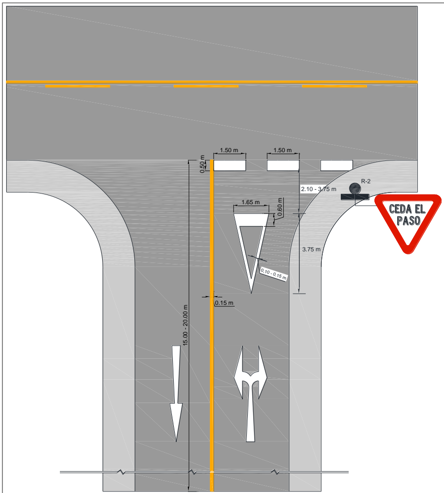
Figura 3.34 Dimensiones de demarcación "CEDA EL PASO"
