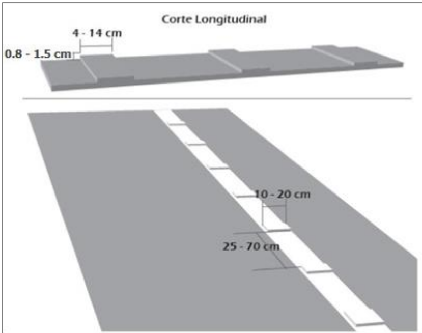
Figura 3.56 Ejemplo de demarcación resaltada
