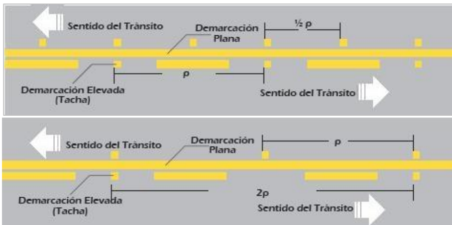
Figura 3.7 Ejemplo de líneas combinadas o mixtas
