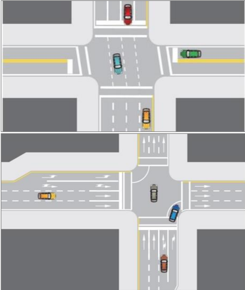
Figura 3.5 Ejemplo de demarcaciones de continuidad de carriles en intersección
