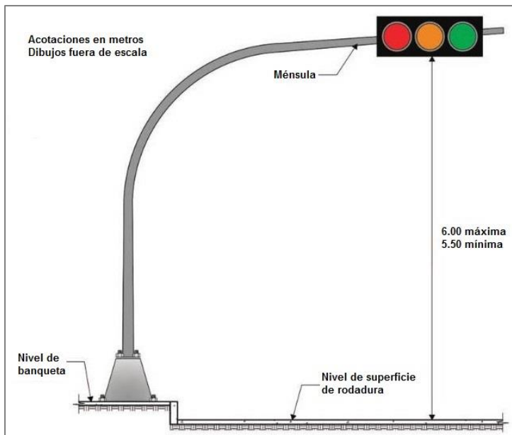
Figura 6.2 Ejemplo de soporte de semáforo tipo ménsula
