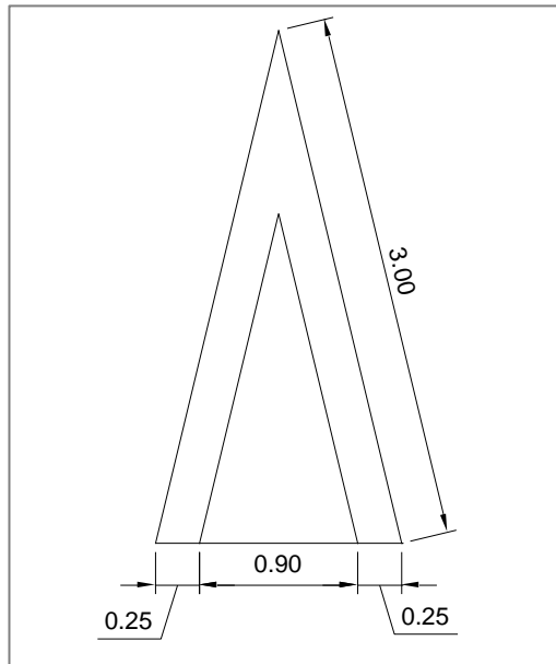
Figura 3.40 Dimensiones de demarcación de "DISTANCIADORES"
