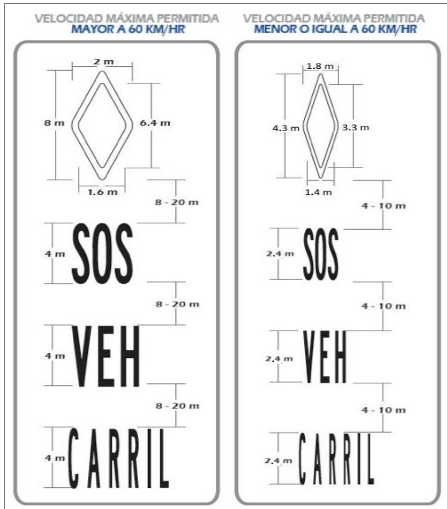
(Continua) Figura 3.42 Ejemplo de demarcación en el pavimento de palabras, símbolos y leyendas
