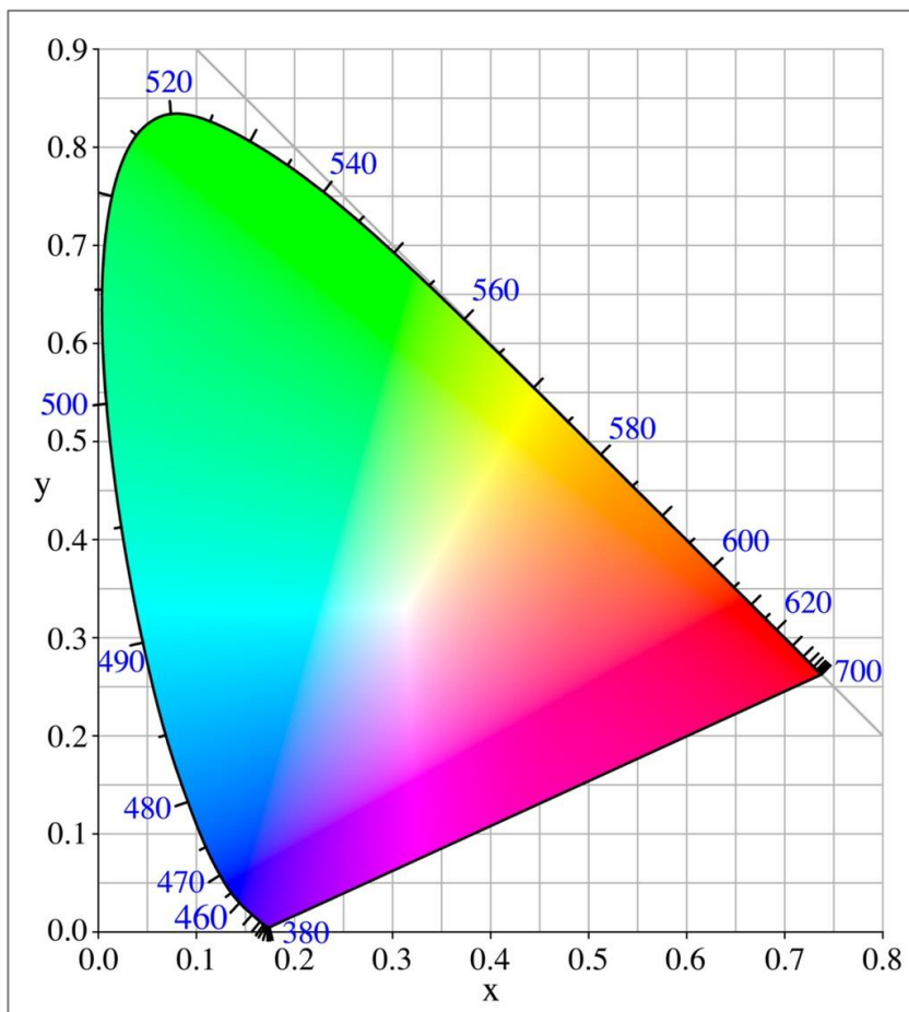
Figura 2.1 Diagrama Cromático CIE 1931
