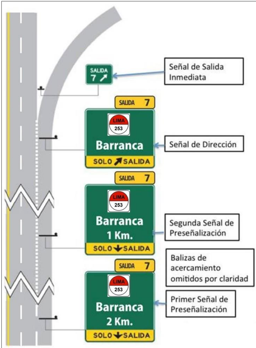
Figura 2.32 Ejemplo de señales de pre señalización en carriles de solo salida o deceleración
