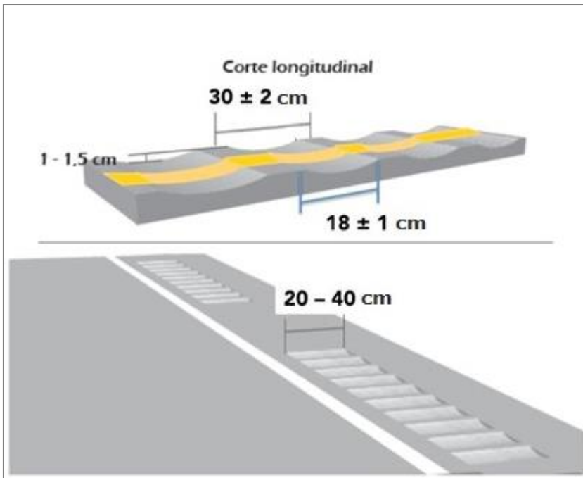
Figura 3.57 Ejemplo de demarcación bajo relieve
