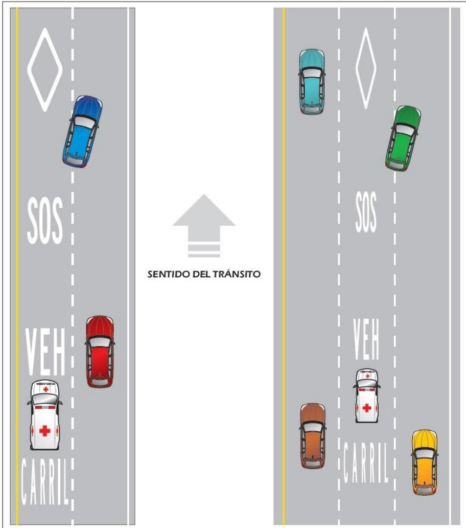
Figura 3.42 Ejemplo de demarcación en el pavimento de palabras, símbolos y leyendas
