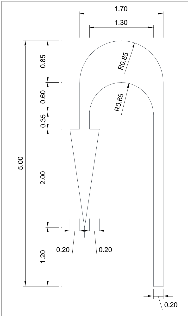
Figura 3.48 Dimensiones de flecha de giro en "U" (m)
