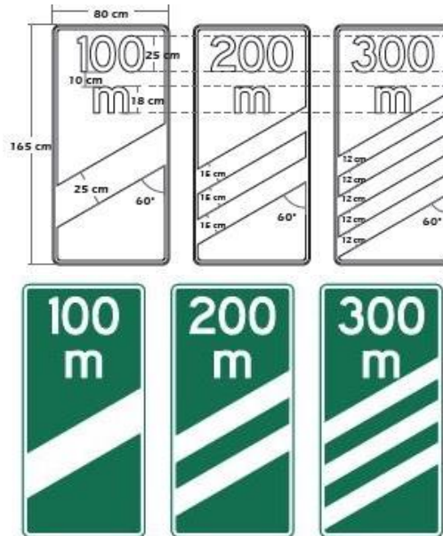
Figura 2.36 Balizas de Acercamiento
