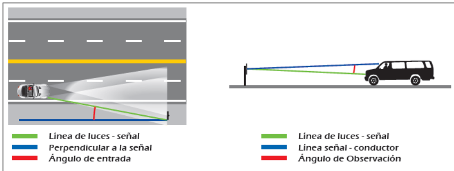
Figura 2.3 Retroreflexión
