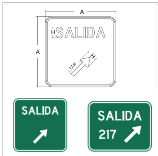
Figura 2.37 Ejemplo de señales salida inmediata
