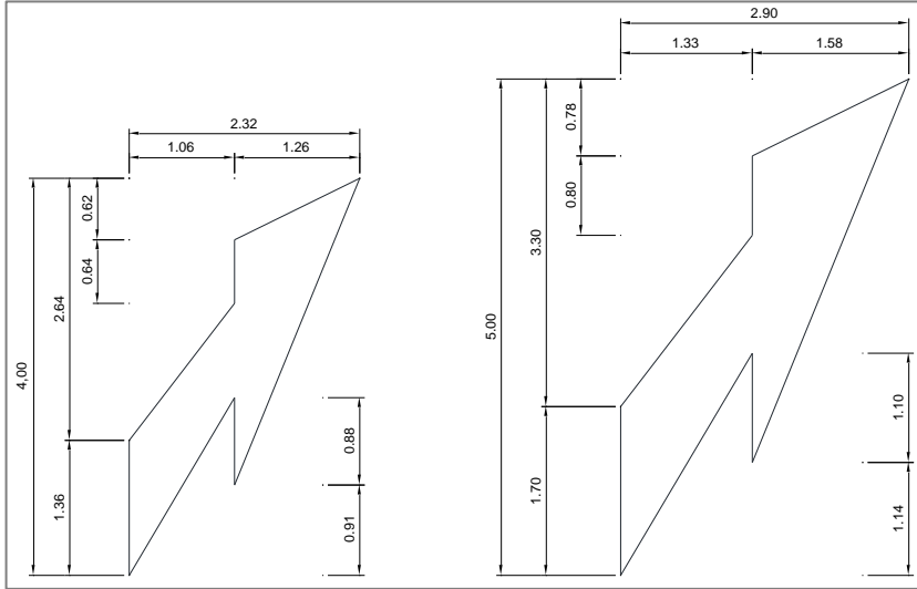
Figura 3.51 Dimensiones de flecha incorporación a carriles exclusivos (m)
