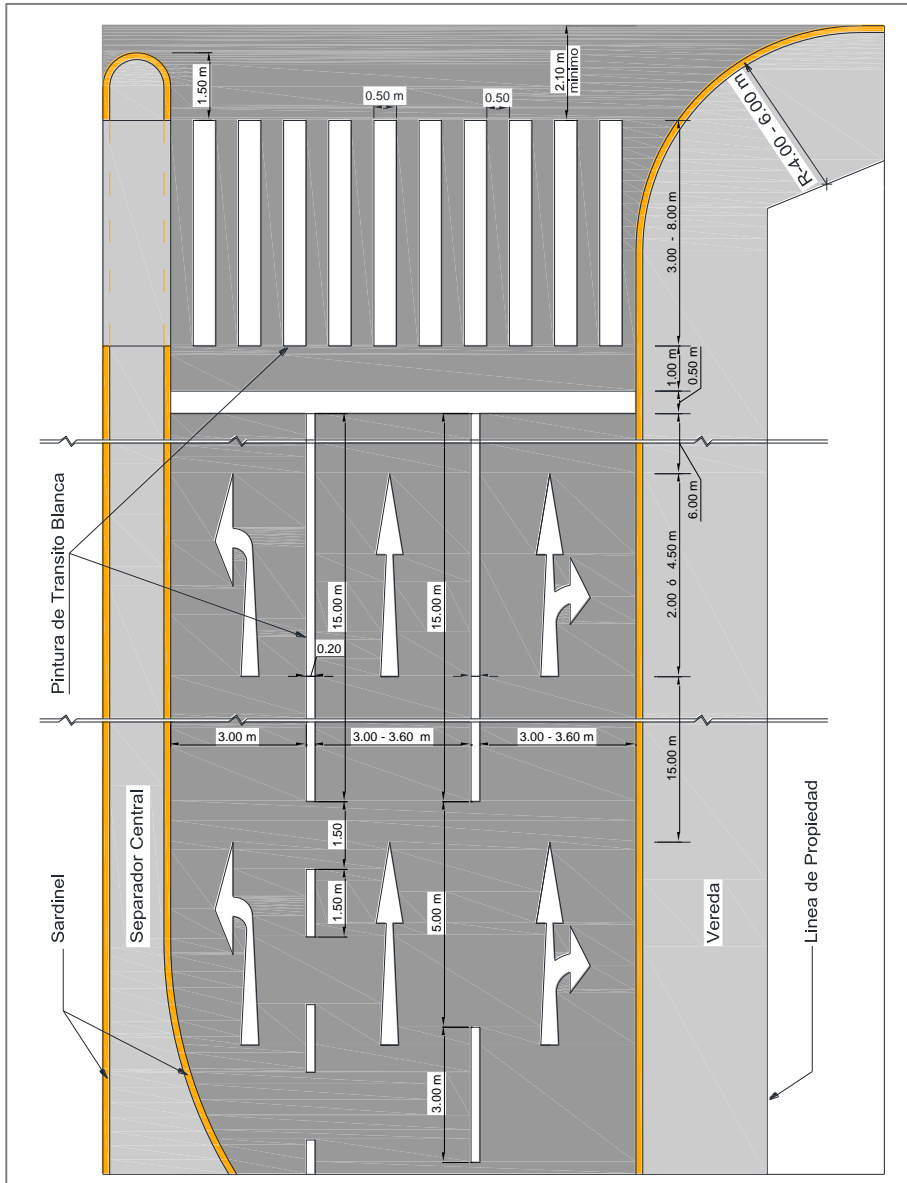
(Continúa) Figura 3.14 Ejemplos de demarcación de línea de pare con dimensiones
