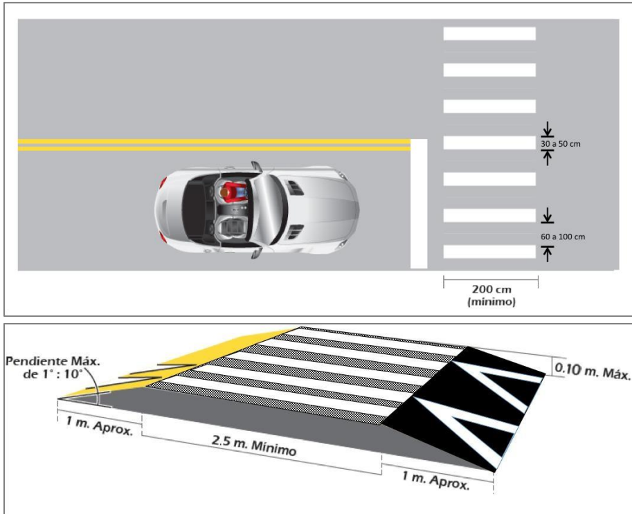
Figura 3.15 Ejemplo de demarcación líneas de cruce peatonal
