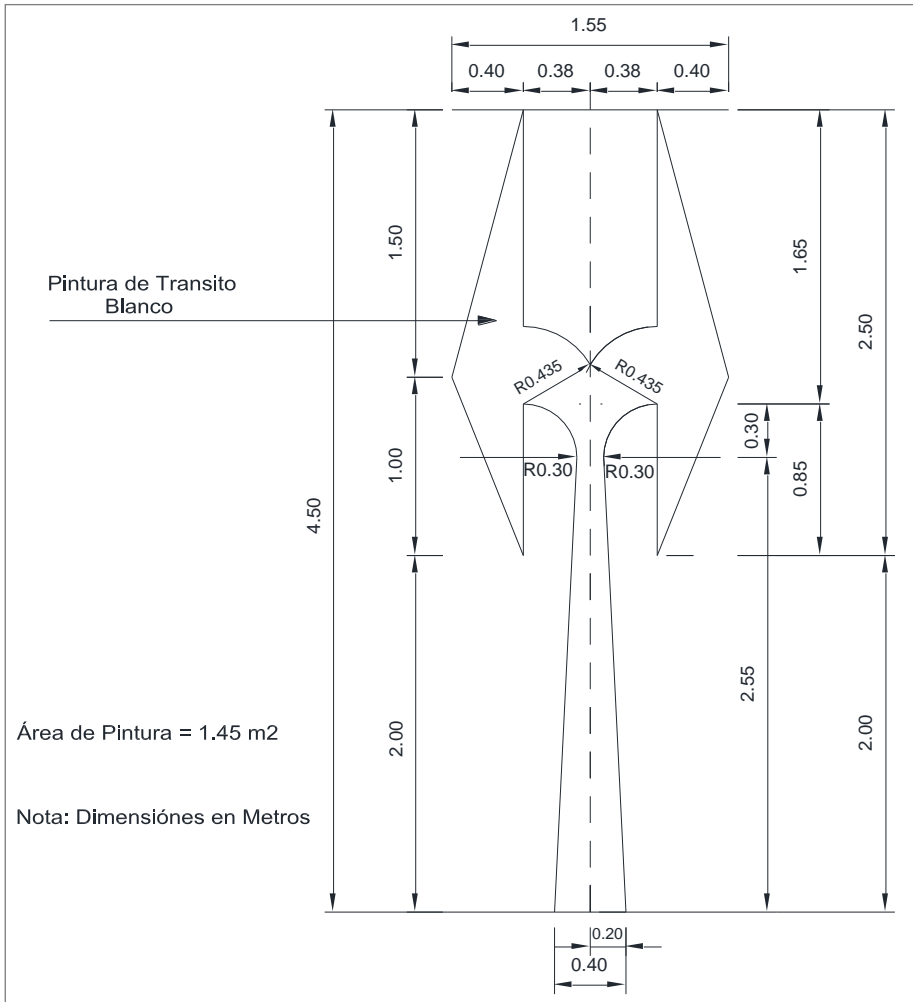
Figura 3.46 Dimensiones de flecha de giro a la derecha e izquierda
