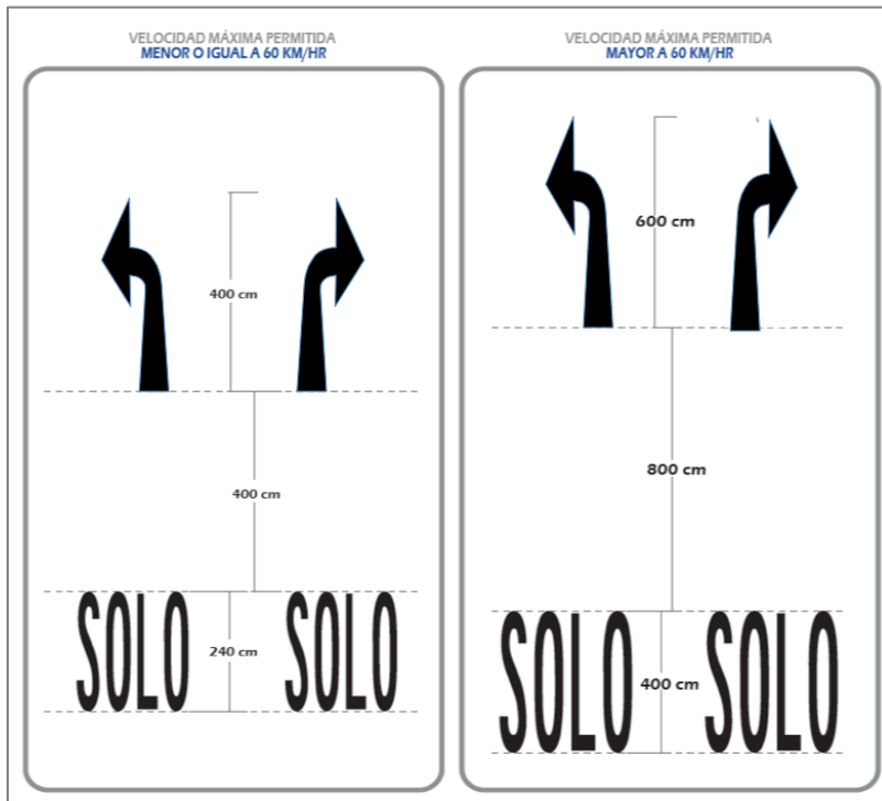
Figura 3.45 Dimensiones de flecha de giro reforzada con la palabra "SOLO"
