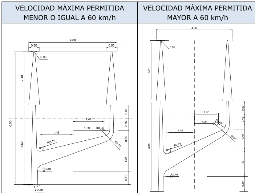
Figura 3.51 Dimensiones de flecha incorporación a carriles exclusivos (m)
