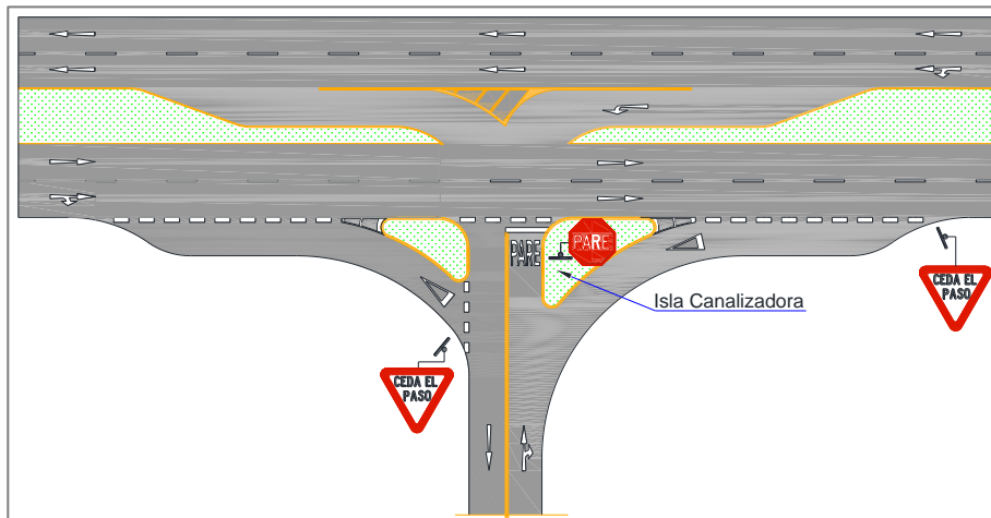
Figura 3.11 Ejemplo de demarcación en el pavimento en una intersección a nivel con islas canalizadoras
