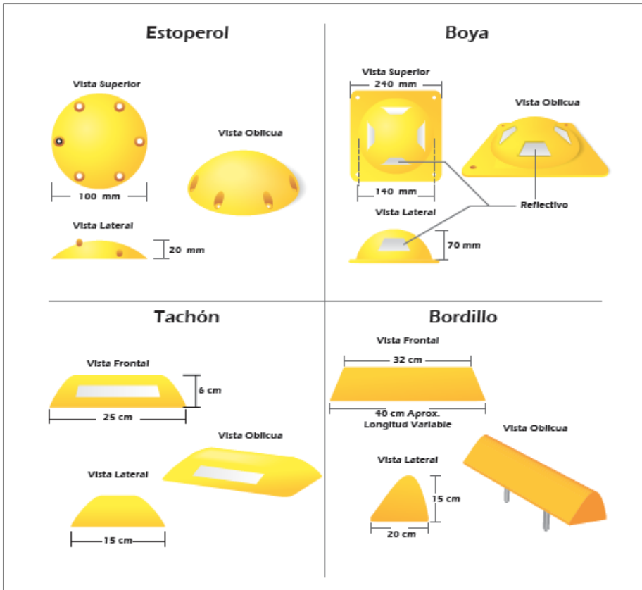
Figura 3.55 Ejemplos de otros delineadores de piso
