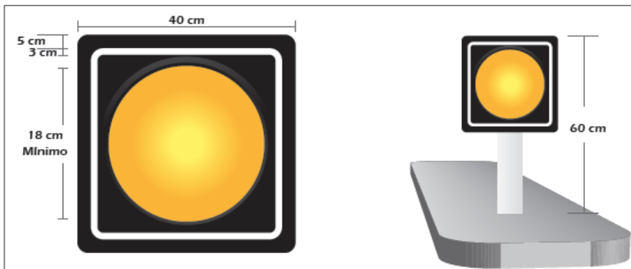
Figura 3.70 Ejemplo y dimensiones de delineadores con luces
