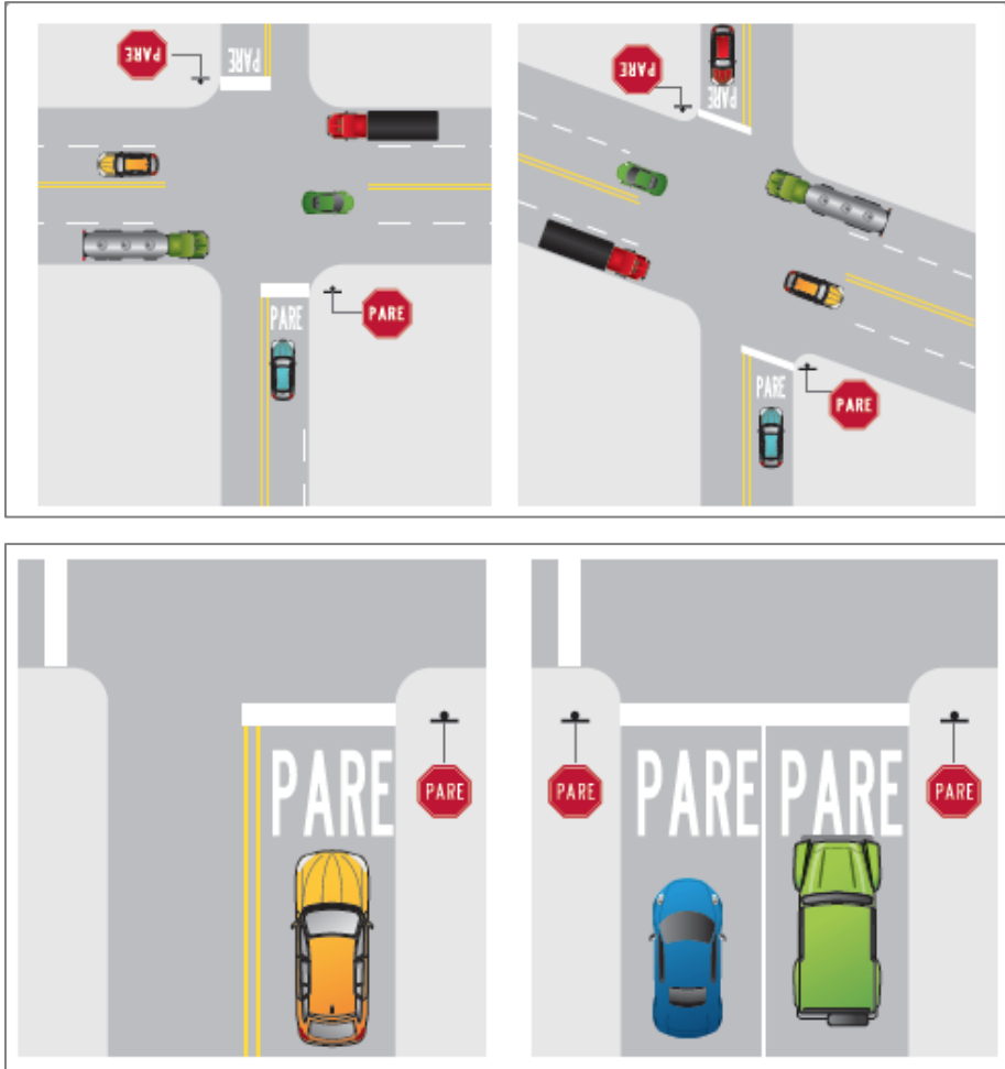
Figura 3.14 Ejemplos de demarcación de línea de pare
