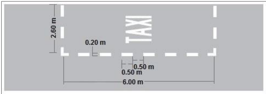
Figura 3.17 Ejemplo de demarcación de estacionamiento para servicios de taxi
