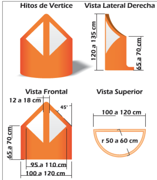
Figura 5.10 Ejemplo de hitos de vértice con dimensiones
