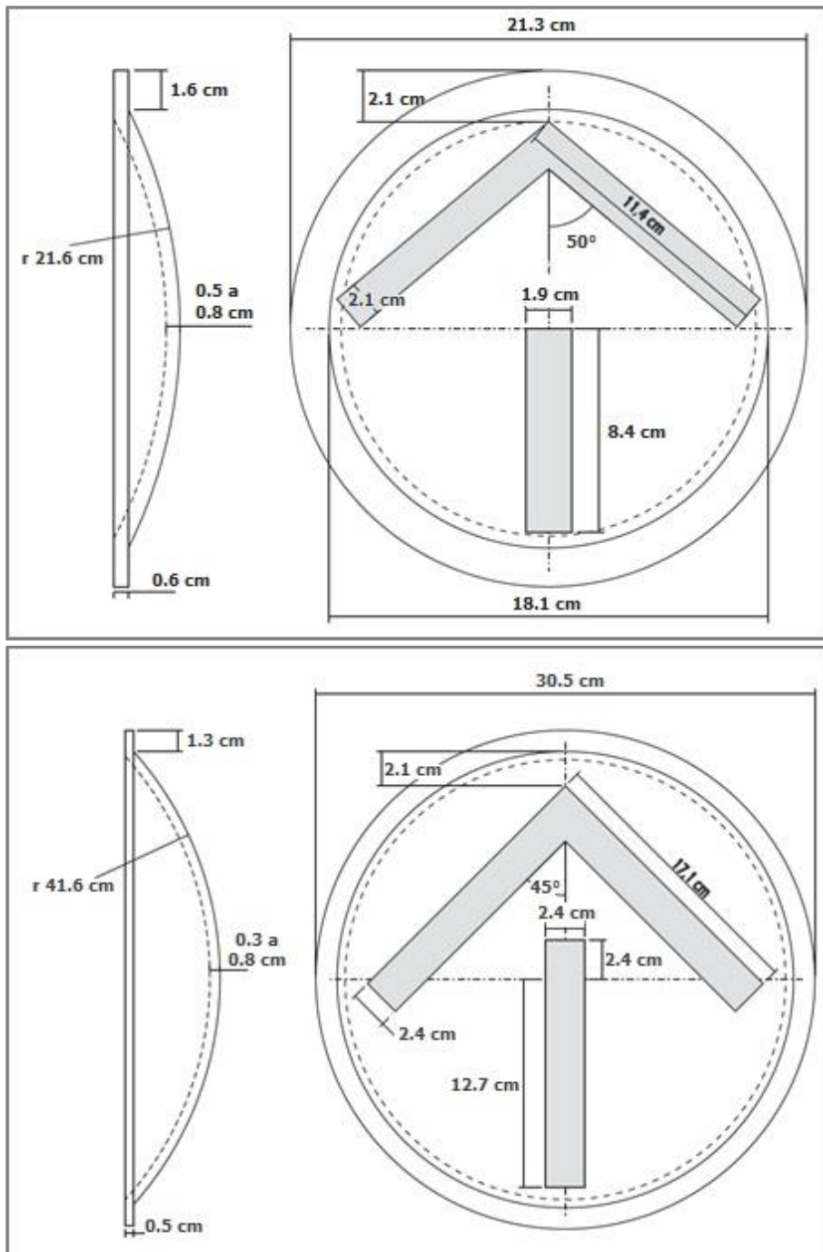
Figura 6.9 Ejemplo de lentes de 0.20 y 0.30 m
