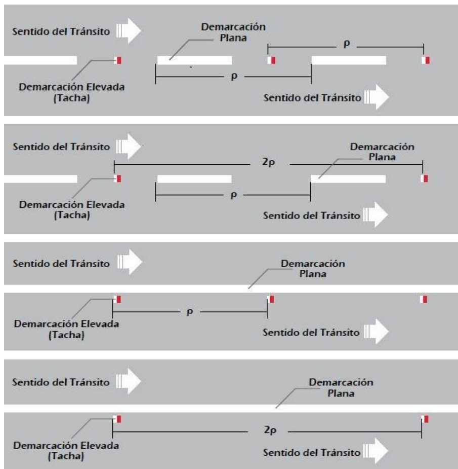
Figura 3.4 Ejemplos de línea de carril segmentada
