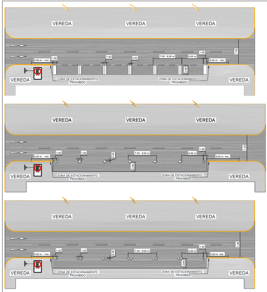
Figura 3.16 Ejemplos de demarcación en espacios para estacionamiento de vehículos con dimensiones
