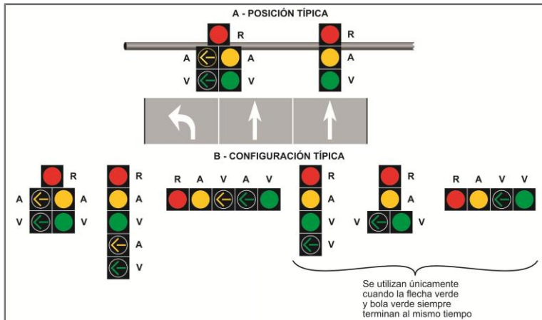
Figura 6.29 Ejemplo de disposición de indicadores de semáforos para giros a la izquierda protegidos y permitidos
