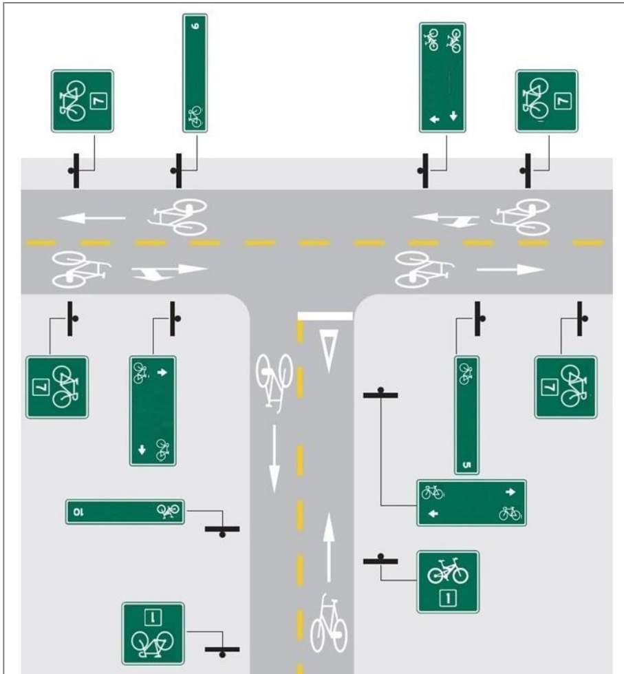
Figura 4.4 Ejemplo de aplicación de una señalización en una intersección de "CICLOVÍAS".
