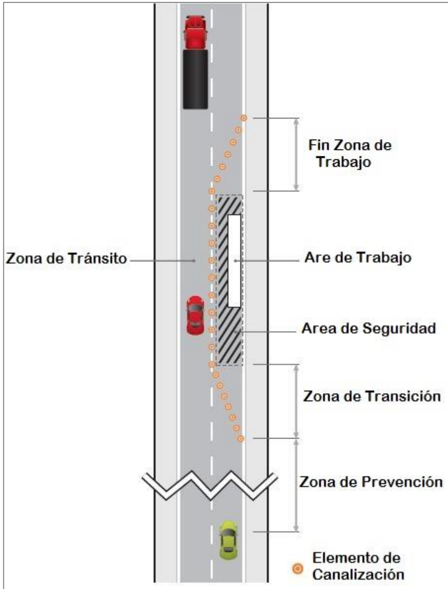
Figura 5.1 Ejemplo de una zona de trabajo
